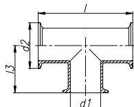
TE CL/CL/CL TEE CL/CL/CL TE CL/CL/CL
