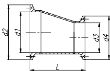
REDUC.EXCÉNTRICA CL/CL EXCENTRIC REDUCER CL/CL REDUCTION EXCEN. CL/CL
