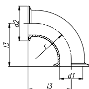
CODO 90° CL/CL BEND 90° CL/CL COUDE 90° CL/CL
