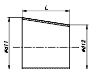
REDUCCIÓN EXCÉNTRICA EXCENTRIC REDUCER REDUCTION EXCENTRIQUE
