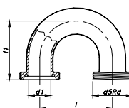
CURVA 180° M/M BEND 180° M/M COUDE 180° M/M
